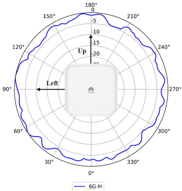
6GHz (Horizontal)
