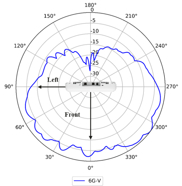
6GHz (Vertical)
